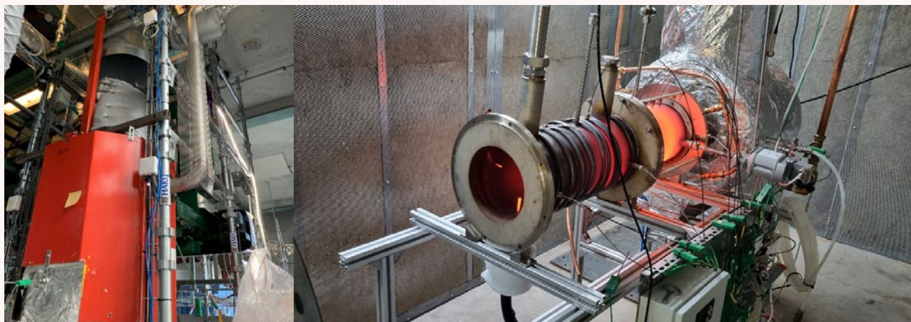
Figur 11: Scarlettriggens där det ingår en förgasare (vänster) gasrening och en brännkammarrigg (höger) där förbränningsprov med förgasad biomassa, gasol kan göras. Riggen nu kompletteras med vätgas och metan för fullständiga prov av prestandan in om BioFlexGen och Biokraft 2023!. Omfattande förgasningsprov ska göras inom EUCANwin!
